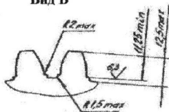
Вид В
